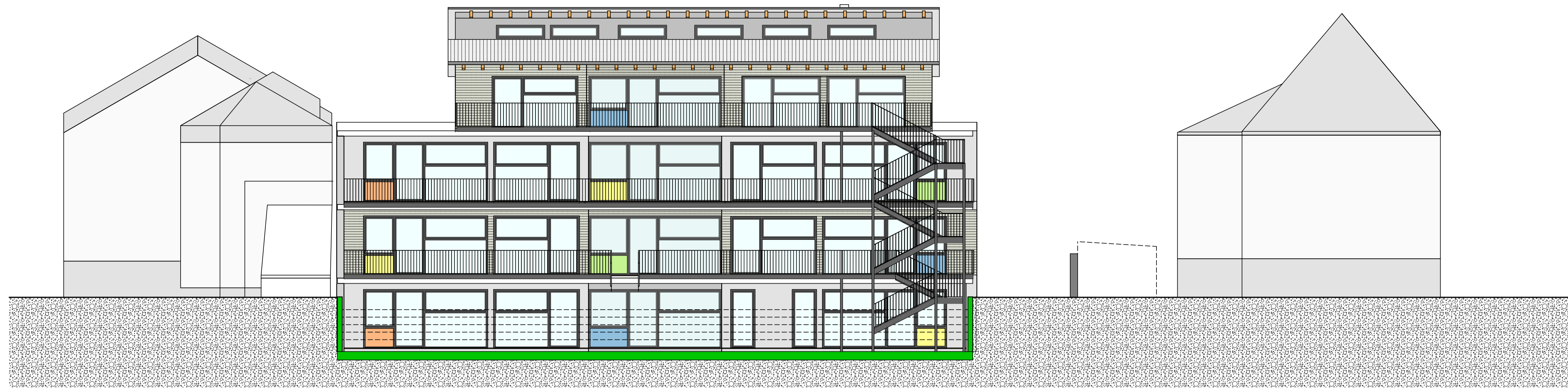
ANSICHT OST
